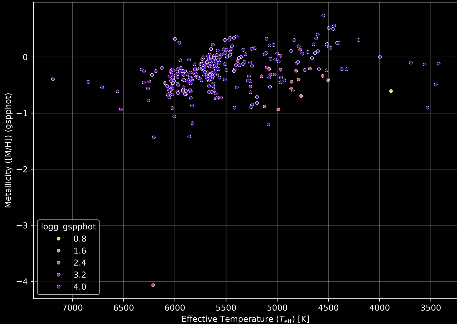
GALAH DR4 Field: [6840] Stellar Population Parameters (n= 287)
