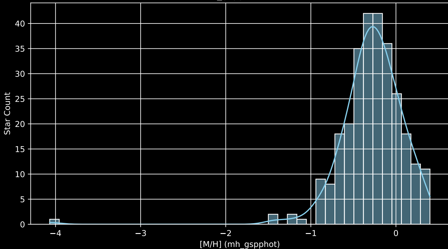
GALAH DR4 Field: [6840] [M/H] (mh_gspphot) (n= 283)
