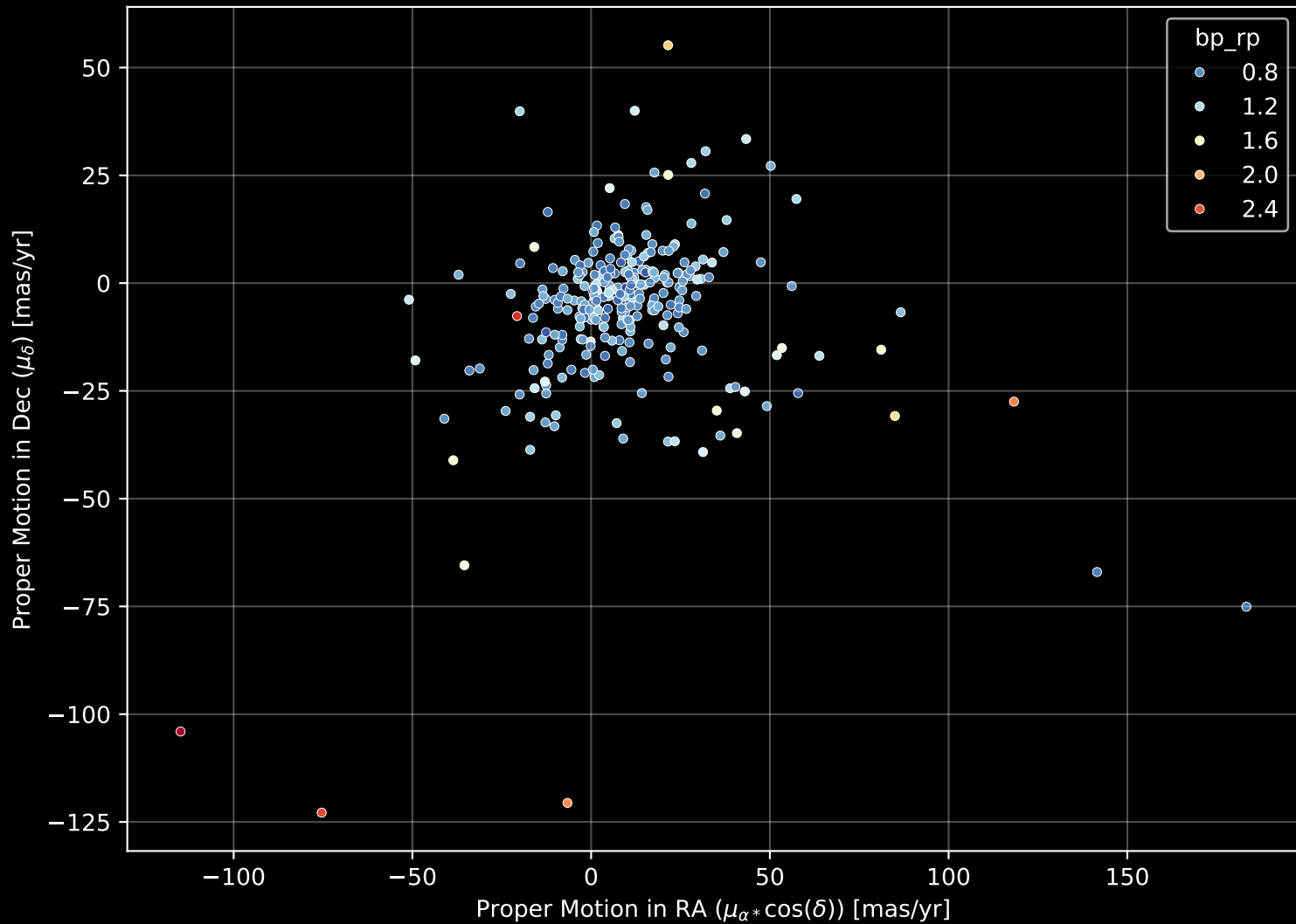
GALAH DR4 Field: [6840] Proper Motion Diagram (n= 287)
